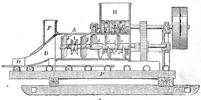
1. Машина Бржовскаго для вырѣзки торфа. 2. Устройство ея ножей: А—планъ, В—боковой видъ. 3. Станокъ для приготовления столоваго торфа. 4. Устройство пробителя въ машинѣ Шликейзена. 5, 6 и 7. Плавы, поперечный и продольный разрѣзы машинъ для прессованія торфа Шликейзена.
