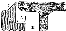
14. Жестяной наугольник (1—разрѣзъ металлической пластинки. 2—стенка улья. 3—жестяной наугольникъ на беруисьмъ грабъ рамки).
