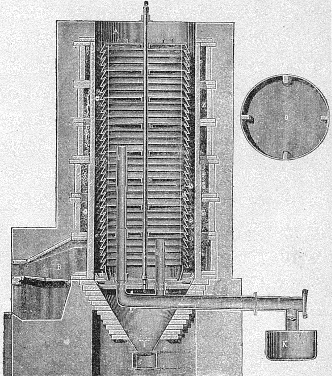
3. Стоячая реторта Родле для коксованія бурого угля и торфа.
