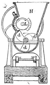
1. Машина Бржовскаго для вырѣзки торфа. 2. Устройство ея ножей: А—планъ, В—боковой видъ. 3. Станокъ для приготовления столоваго торфа. 4. Устройство пробителя въ машинѣ Шликейзена. 5, 6 и 7. Плавы, поперечный и продольный разрѣзы машинъ для прессованія торфа Шликейзена.
