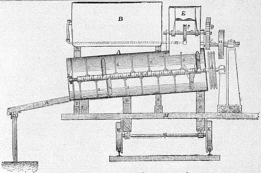
1. Машина для наливного формованного торфа.
