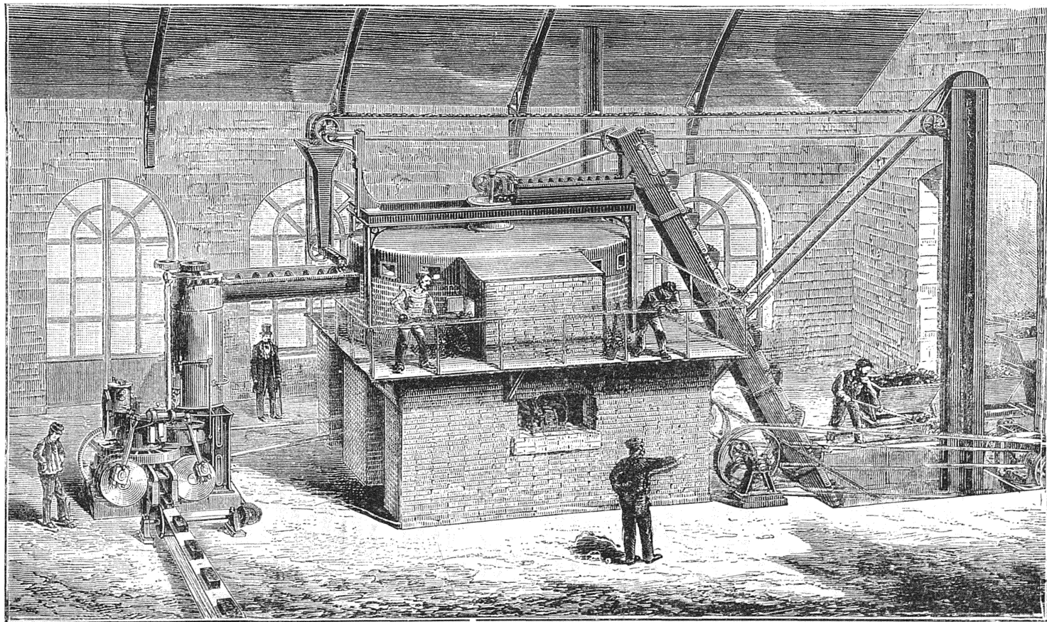
Общий вид устройства для производства угольных брикетов.
