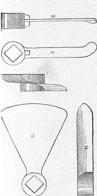
2. Ножи машины для наливного формованного торфа.
