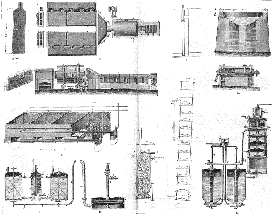
1 Шпатель 2 Гребень 3 Вращающаяся содовая печь съ двумя временами для выпаривания шелока въ огонь (горизонтальный разръзъ) 4 Ома жс (внѣшній видъ) 5 Аппаратъ Дилова Шанкса для вымачиванія содоваго плава 6 Схема устройства въ нѣтъ первушихъ трубъ 7 Подочный хвостъ Гельма для удерживанія сырого содоваго шелока нижнимъ огнемъ 8 Абсорберъ Сольева для насыщанія раствора поваренной соли аммиакомъ 9 Печь для обжиганія извести 10 Карбонизацiонная башня Сольера 11 Вакуумъ-фильтръ для отщепанія кислотъ У соли отъ маточнаго раствора 12 Кальцимировская печь Сольера для кислотъ У соли 13. Генераторъ для аммиака Сольера
